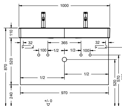
WWLO097 passend zu 235310 mit H2
