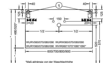
*Maß abhängig von der Waschtischhöhe
