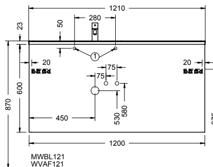
MWBL121 WVAF121 linke Version abgebildet, rechte Version spiegelbildlich
