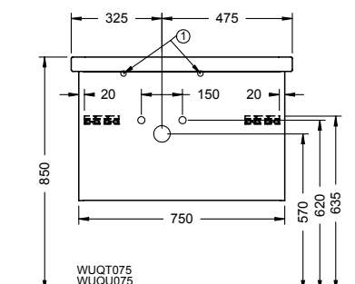
WUQT075 WUQU075 zu 232580 (zu 232680 spiegelbildlich)
