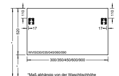
*Maß abhängig von der Waschtischhöhe
