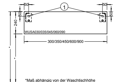
*Maß abhängig von der Waschtischhöhe
