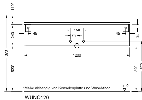
*Maße abhängig von Konsolenplatte und Waschtisch
