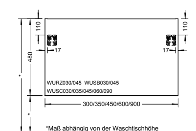
*Maß abhängig von der Waschtischhöhe
