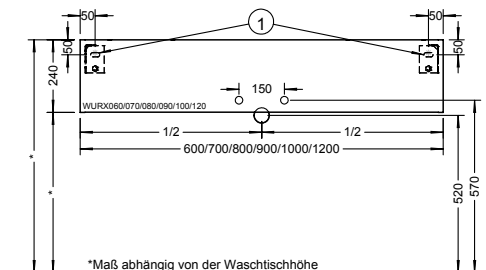
*Maß abhängig von der Waschtischhöhe
