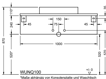
*Maße abhängig von Konsolenplatte und Waschtisch
