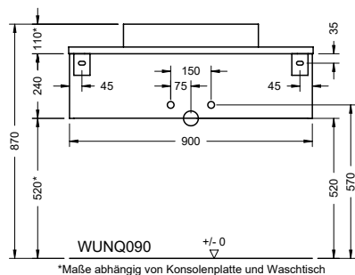
*Maße abhängig von Konsolenplatte und Waschtisch
