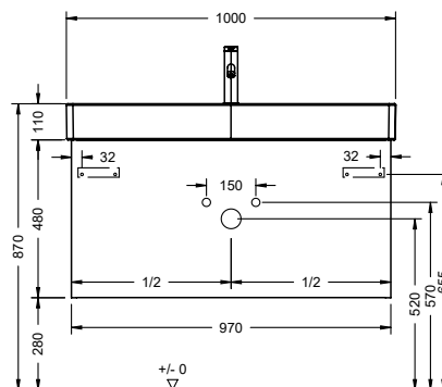
WWLM097 passend zu 235310 mit H1
